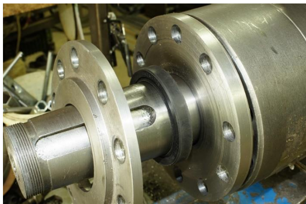
Сальниковое уплотнение
